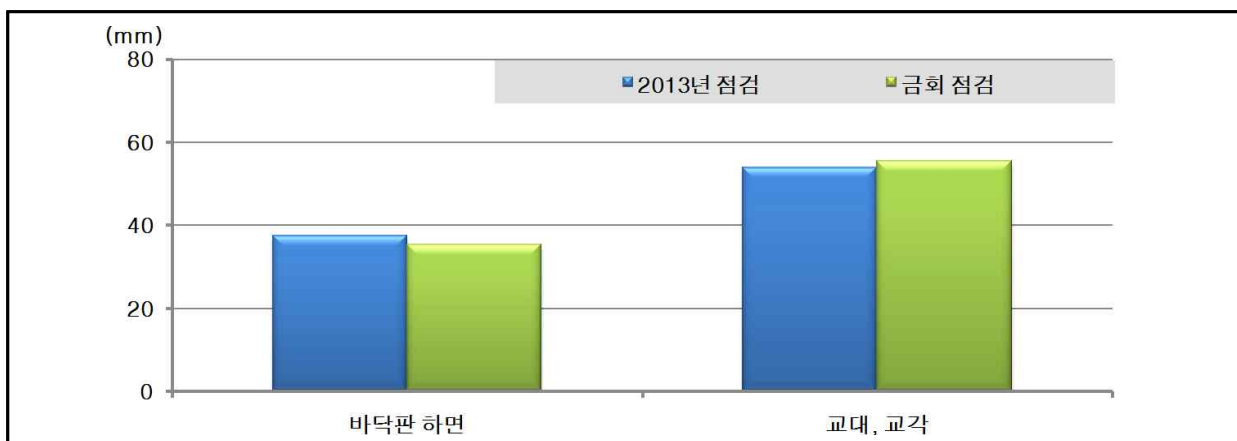
【그림 4.4】 부재별 탄산화깊이에 의한 콘크리트 잔여피복두께 비교
