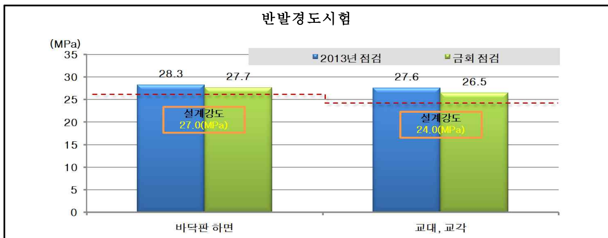
【그림 4.2】 기 점검 자료 비교·분석
